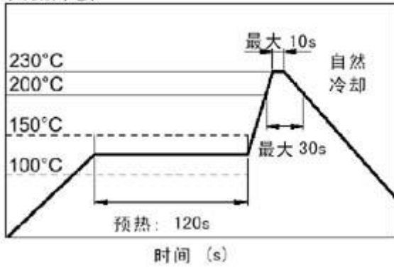
建议焊接条件 回流焊接
